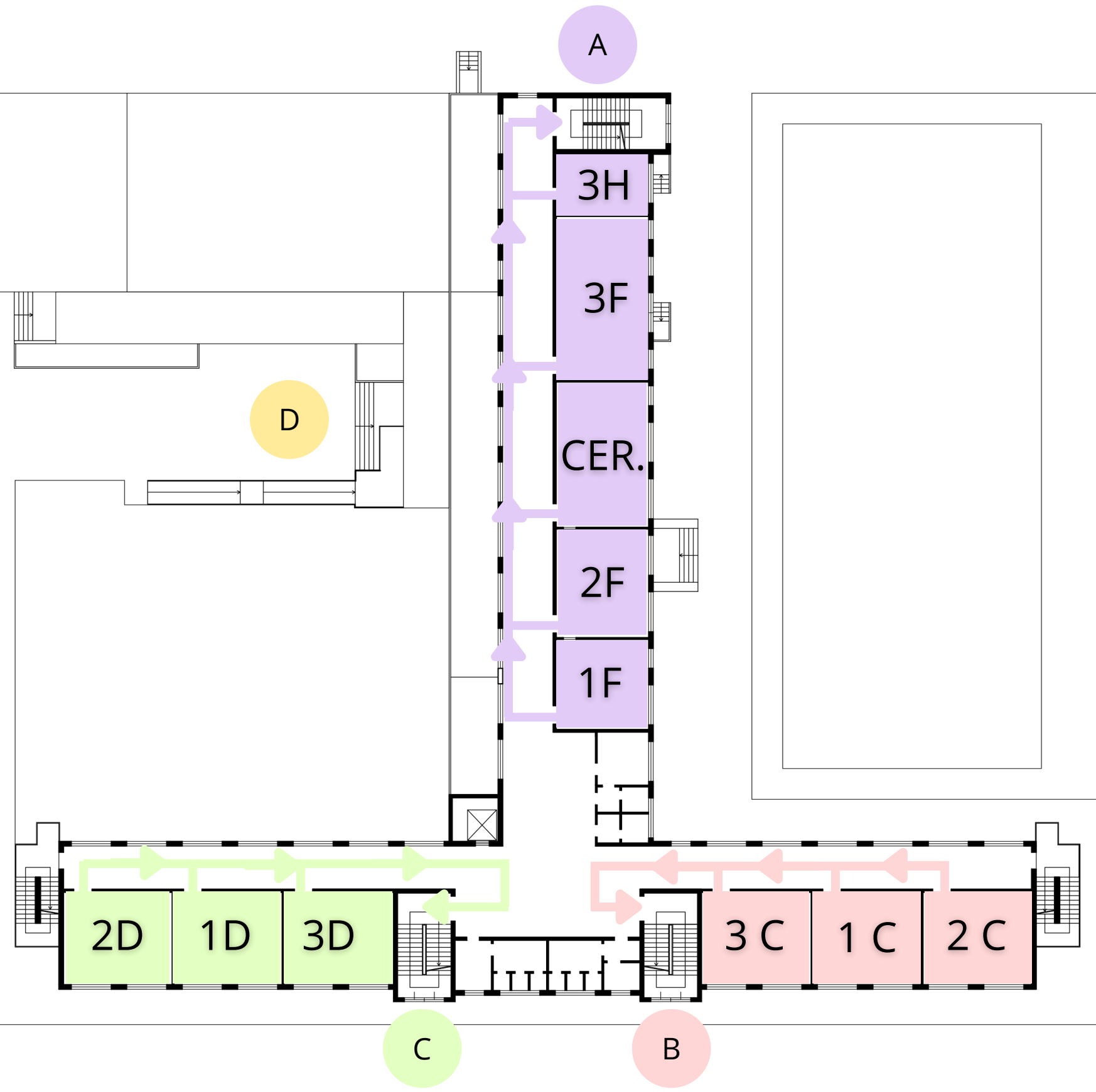
PIANO PRIMO
